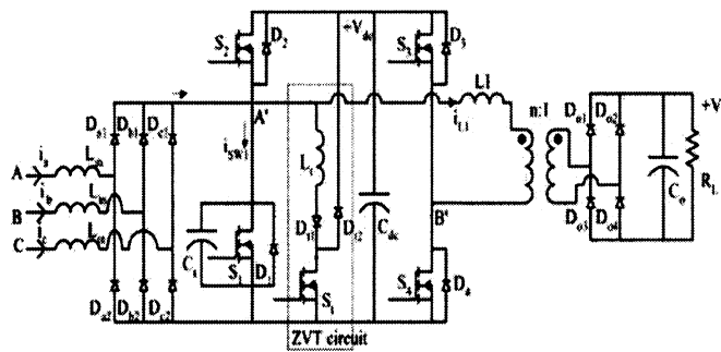
(d) A front-end boost converter technique is used for PFC ([14])
